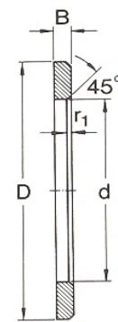
Kroužek s oběžnou drahou - řada LS
