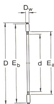
Axiální klec s jehlami řada AXK
