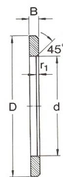
Kroužek s oběžnou drahou - řada LS
