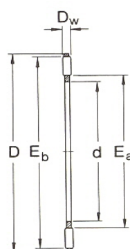
Axiální klec s jehlami řada AXK
