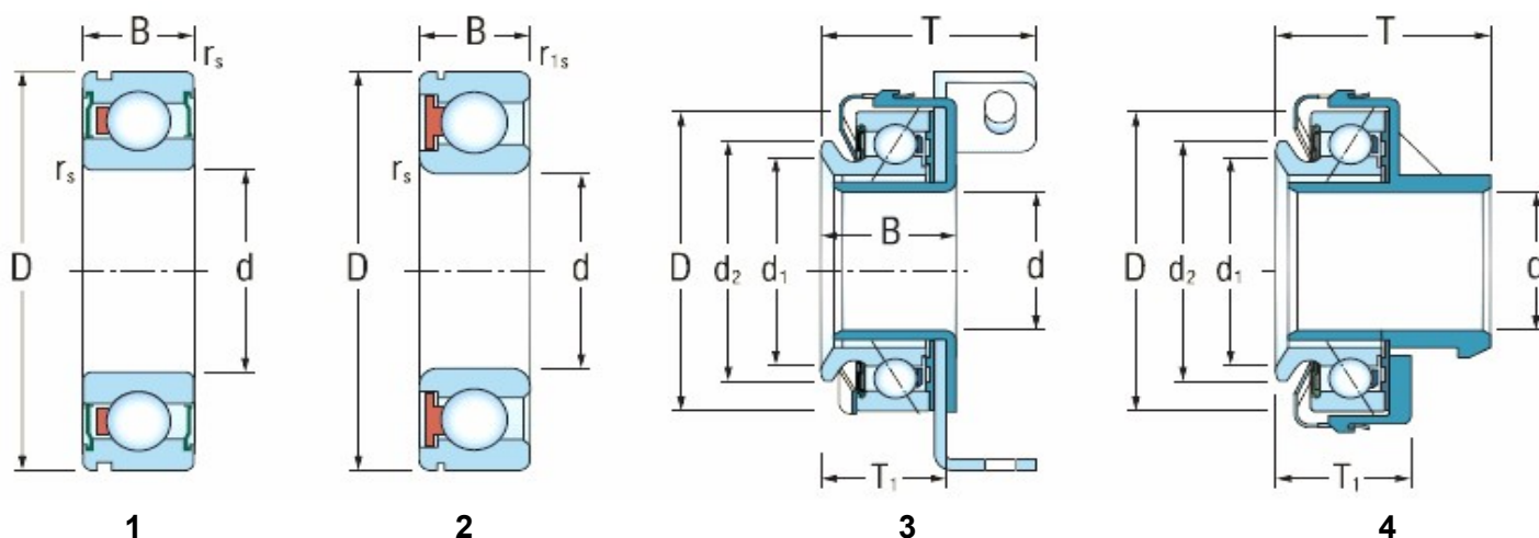
JEDNOŘADÁ KULIČKOVÁ LOŽISKA PLC
