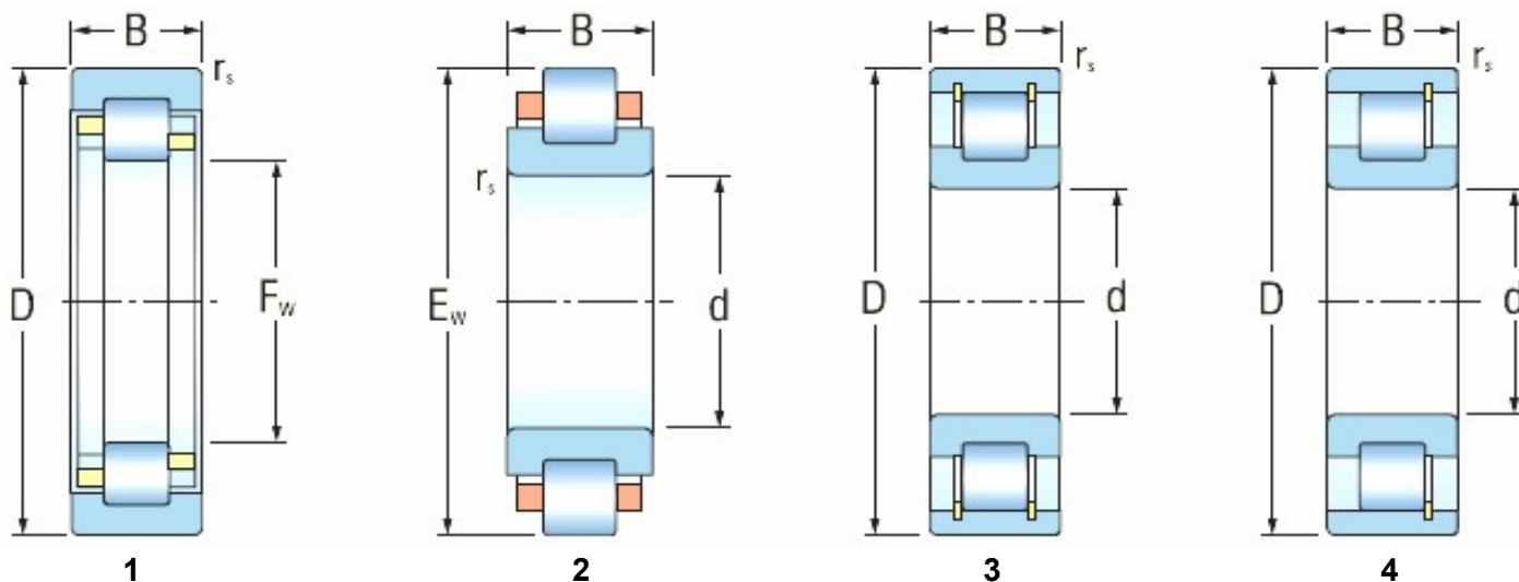
JEDNOŘADÁ VÁLEČKOVÁ LOŽISKA PLC
